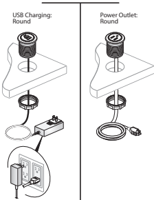
EURT-0072-1100 EURT-0072-1010 Bezel Utility Module
